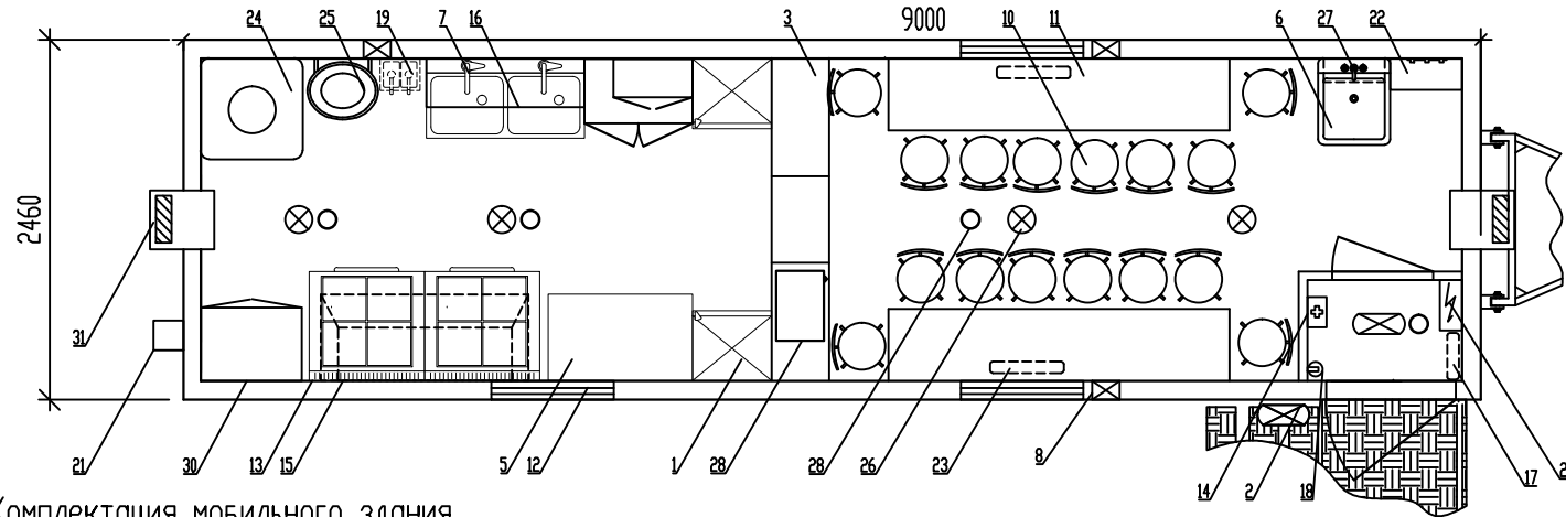
Комплектация мобильного здания
