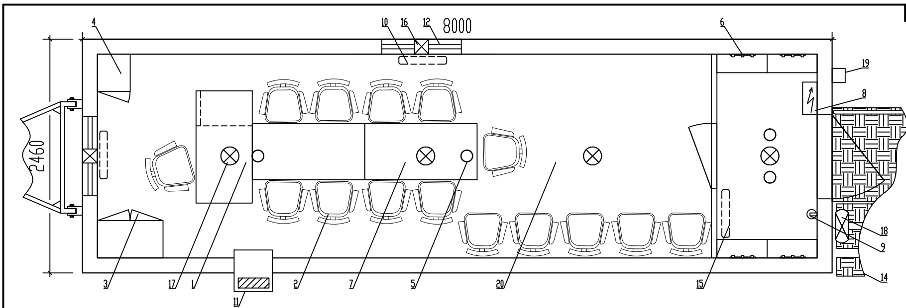
Комплектация мобильного здания
