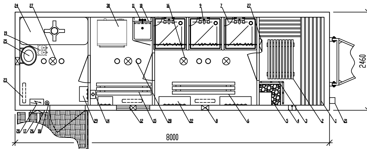
Комплектация мобильного здания
